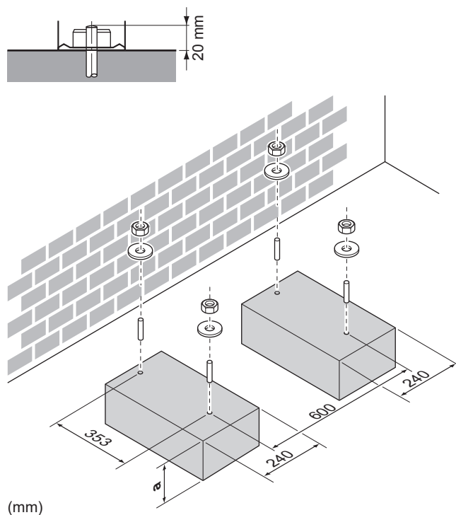
a 100 мм над расчетной поверхностью снежного покрова
