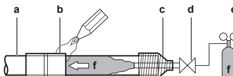
a Трубопровод для хладагента b Припайваемый компонент c Обмотка лентой d Ручной клапан e Редукционный клапан f Азот
